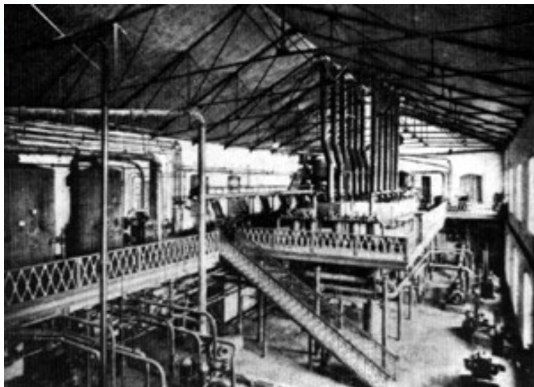
Аппаратный зал Эртильского свеклосахарного завода, построенного Акционерным обществом "Фицнер и Гампер"
