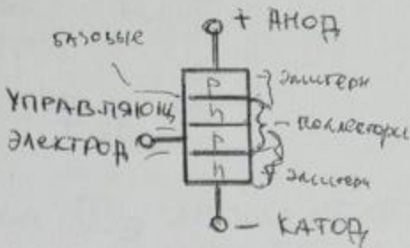
б) триодный
