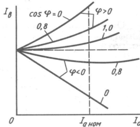
Рис. Внешняя характеристика генератора переменного тока.
