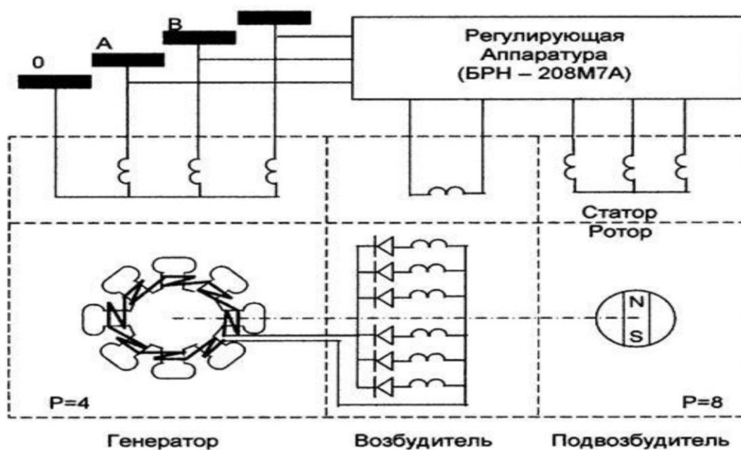
Рис. Структурная схема генератора ГТ-30НЖЧ12.
