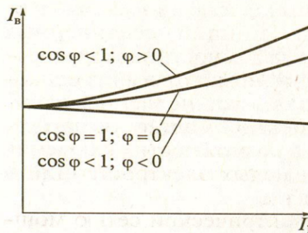
Рис. Регулировочная характеристика генератора переменного тока
